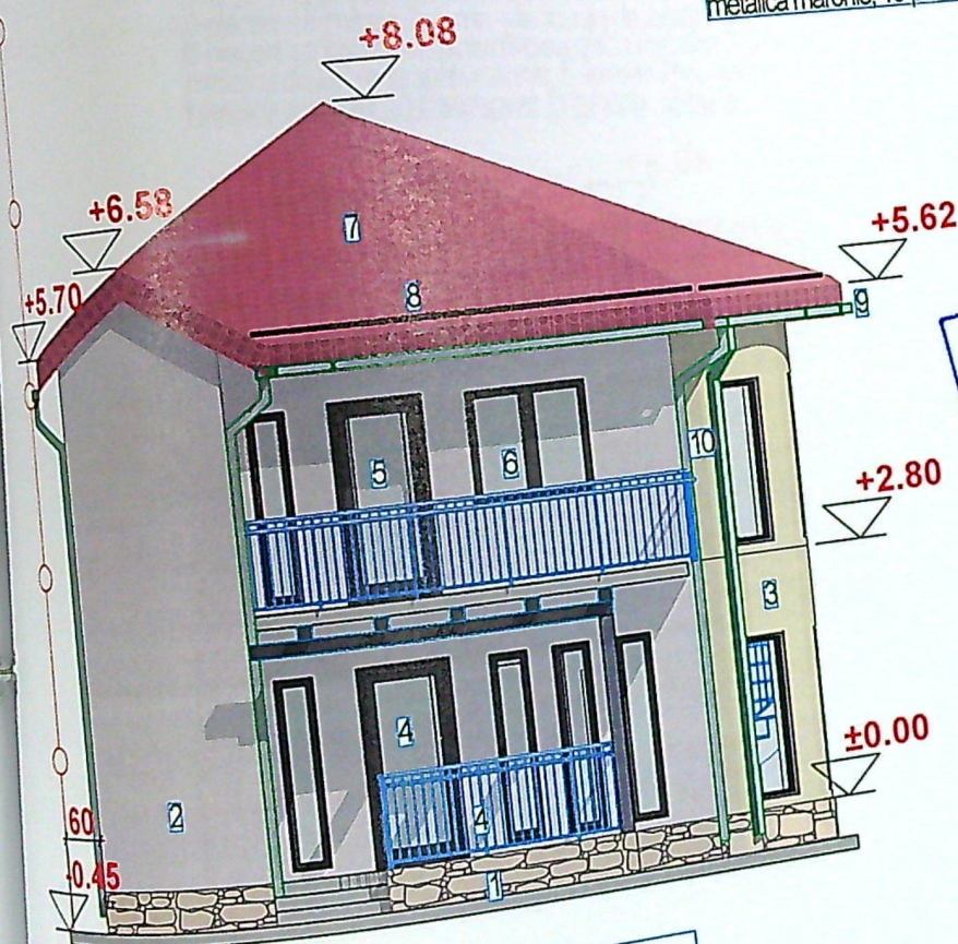
FATADA SECUNDARA
